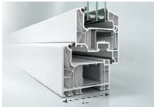
Высокий уровень базовой защиты: увеличенная монтажная глубина профиля и особое расположение фурнитуры затрудняют доступ к элементам запирания.
